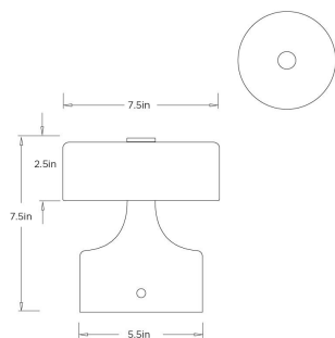
PAC11 VERGLAS MINI RECHARGEABLE ACCENT LAMP
